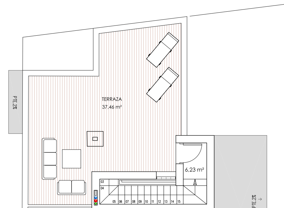
PLANTA CUBIERTA
