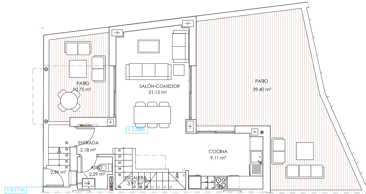
PLANTA BAJA
