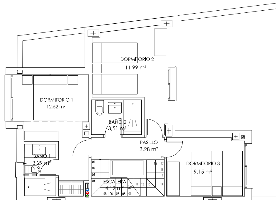
PLANTA PRIMERA
