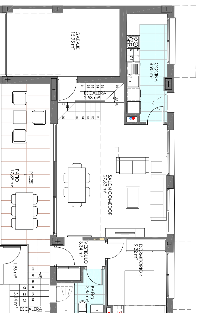
3 PLANTA BAJA
