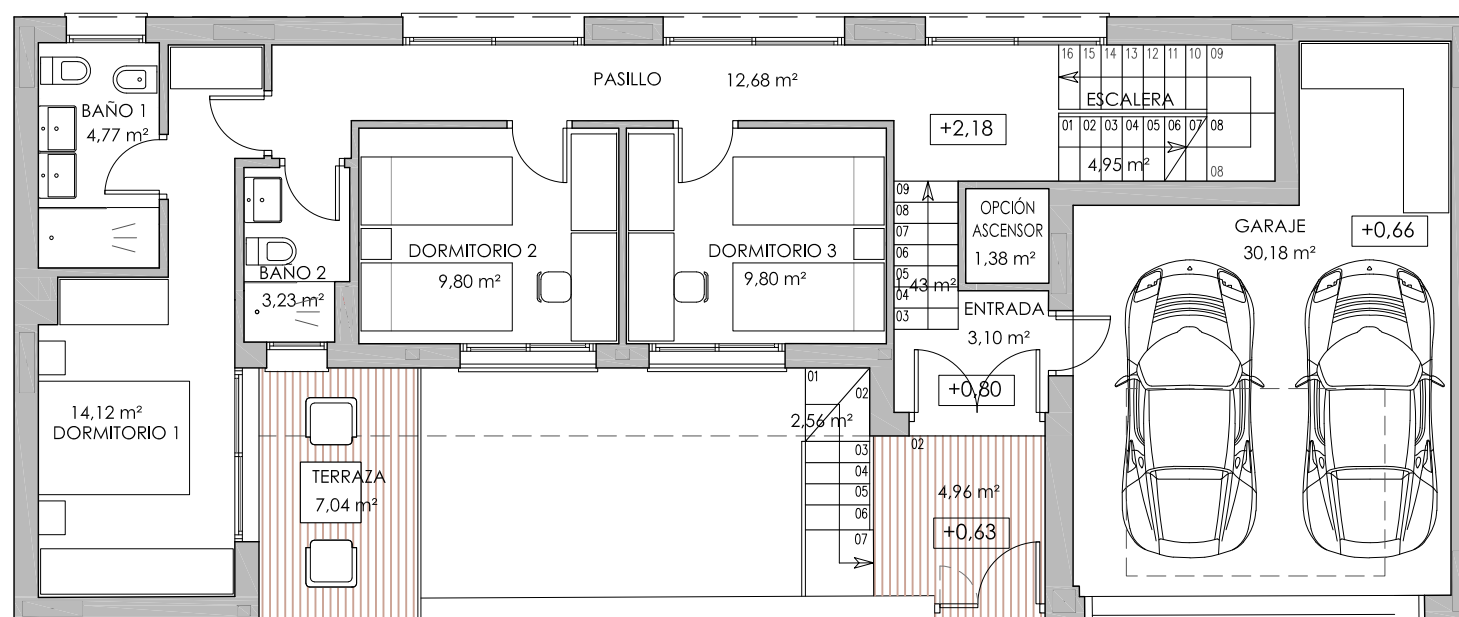
PLANTA BAJA
