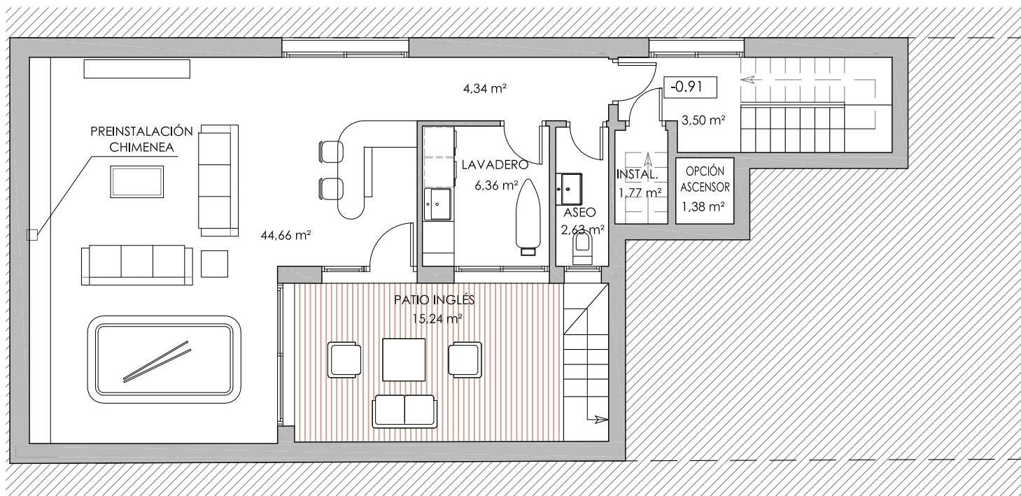
PLANTA SEMISÓTANO
