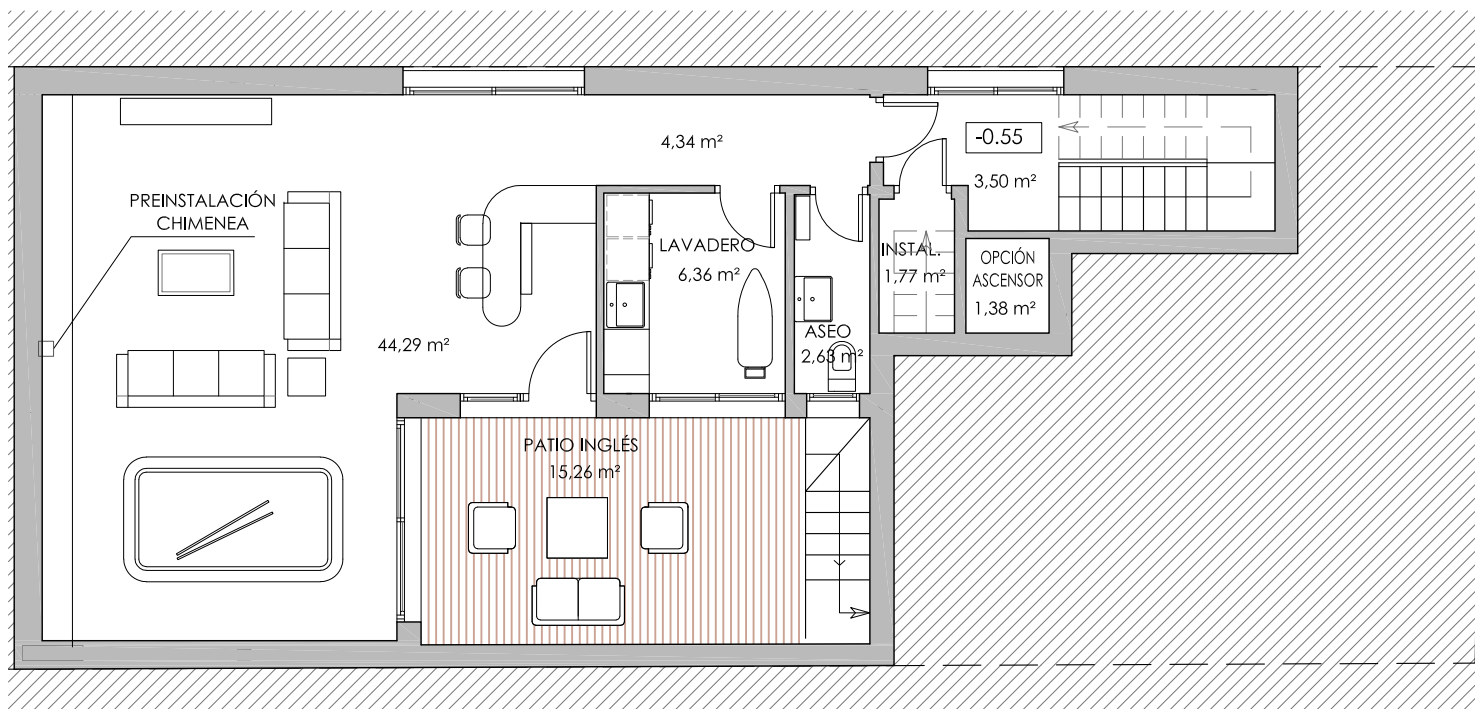
PLANTA SEMISÓTANO
