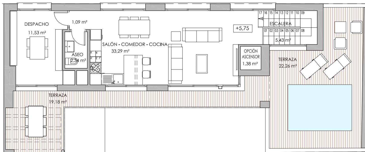
PLANTA PRIMERA
