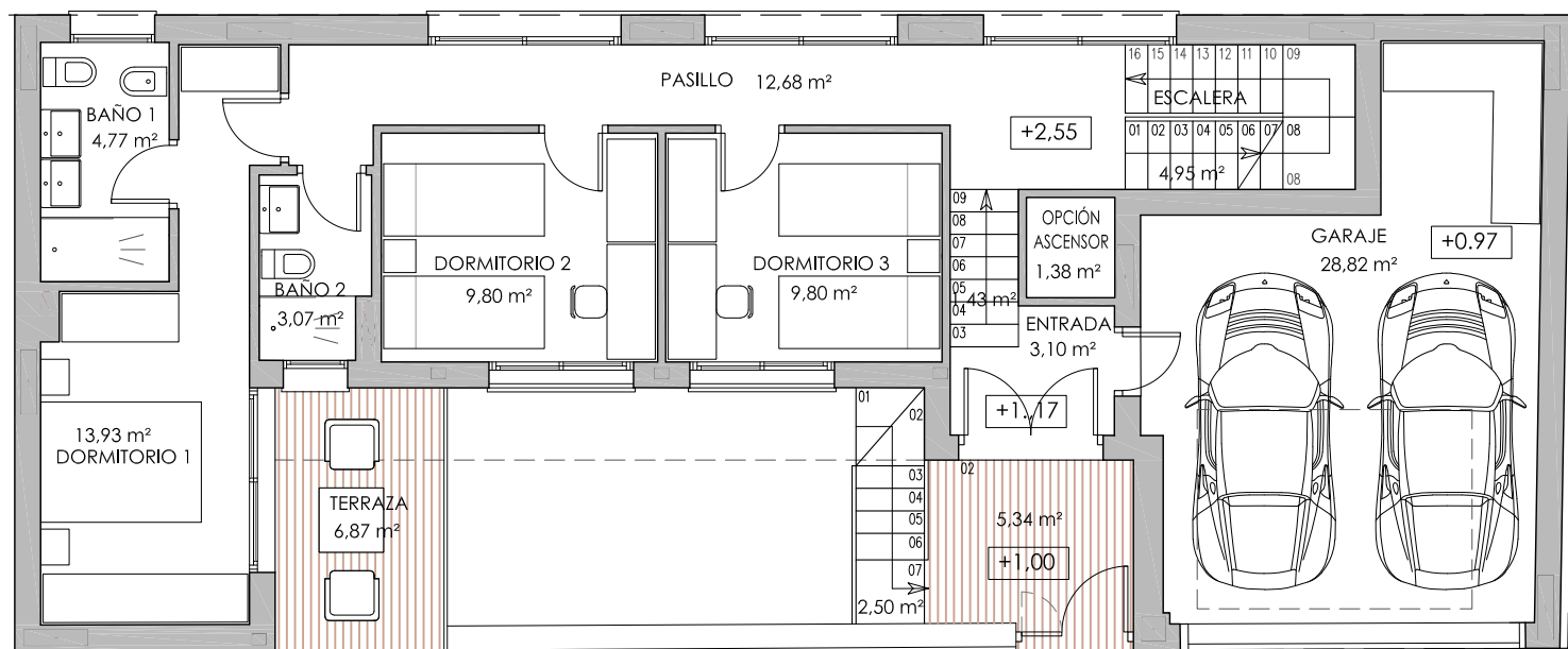
PLANTA BAJA
