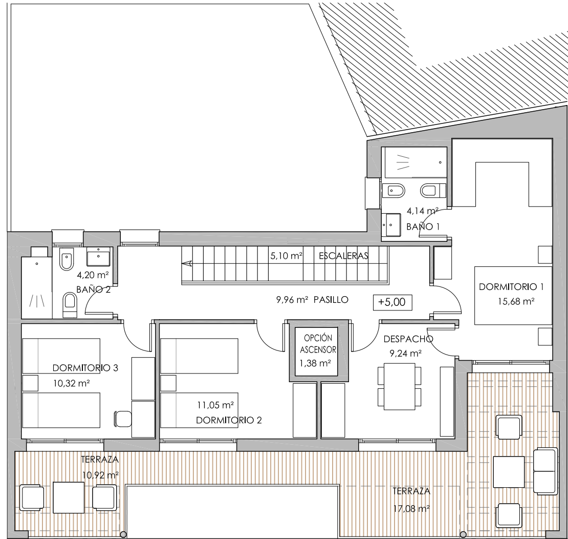
PLANTA PRIMERA
