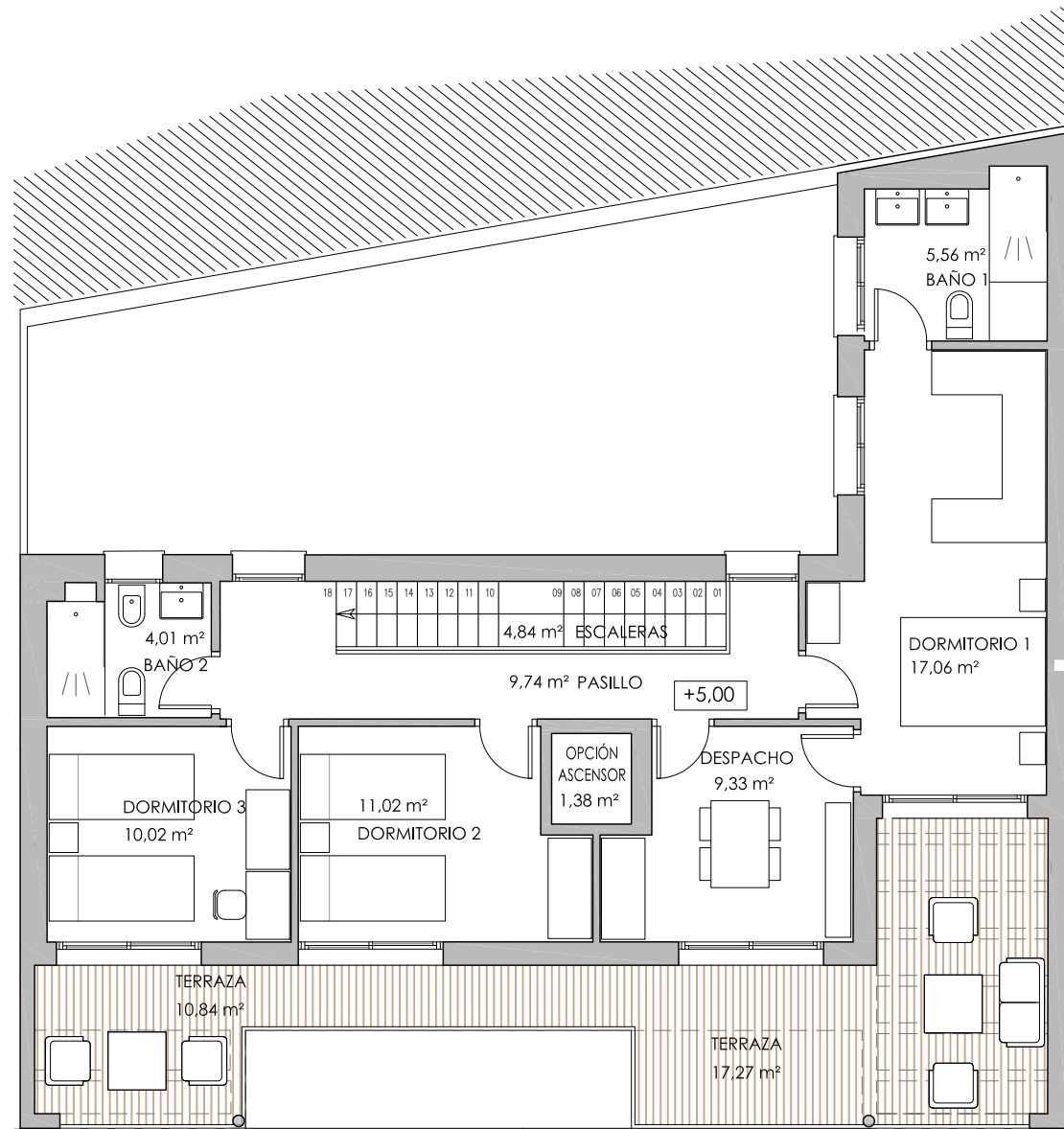
PLANTA PRIMERA
